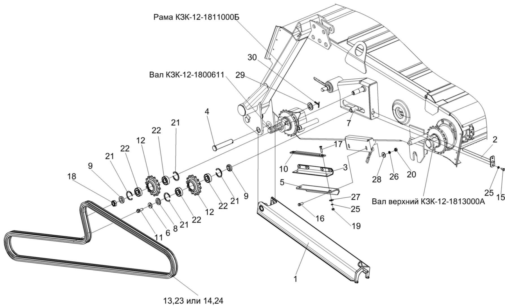
Рисунок 24а – Камера наклонная. Привод транспортера
