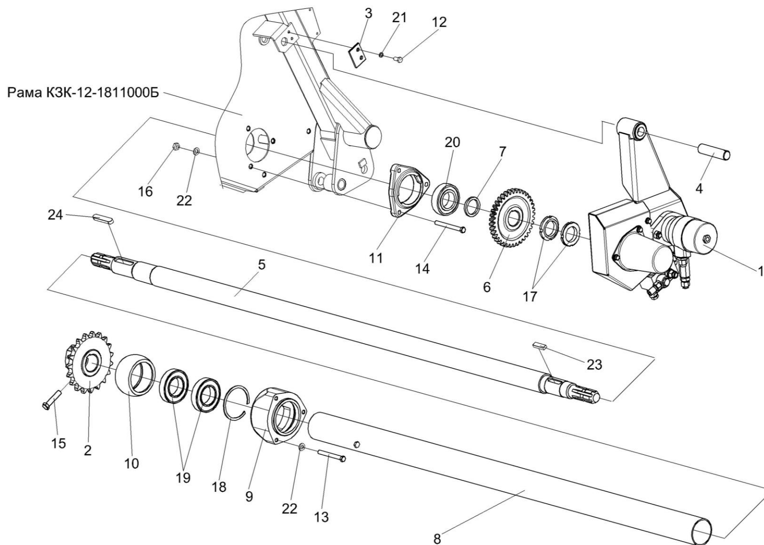
Рисунок 18а – Установка вала КЗК-12-1800611
