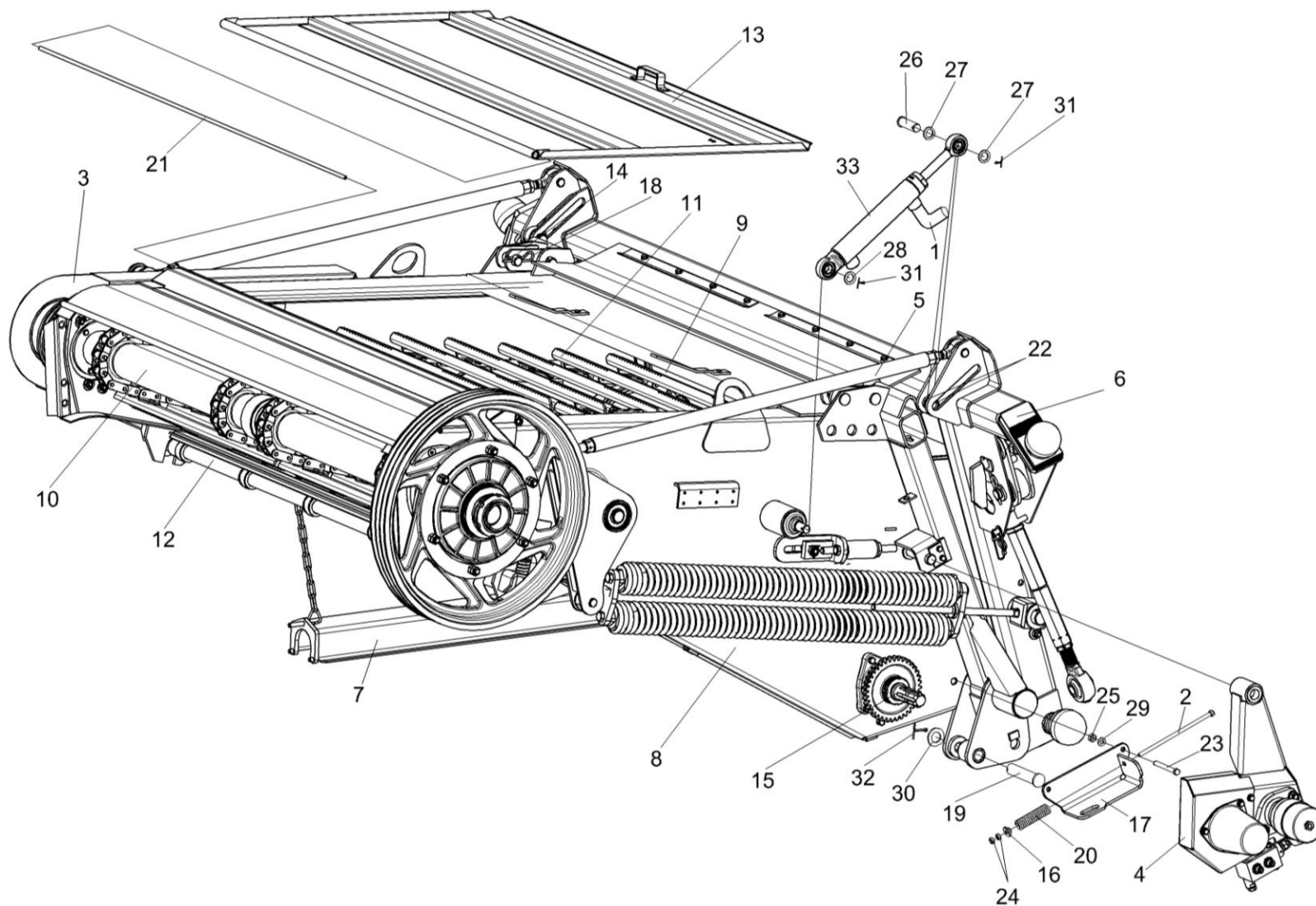
Рисунок 11а – Камера наклонная КЗК-12-1810000Б-01
