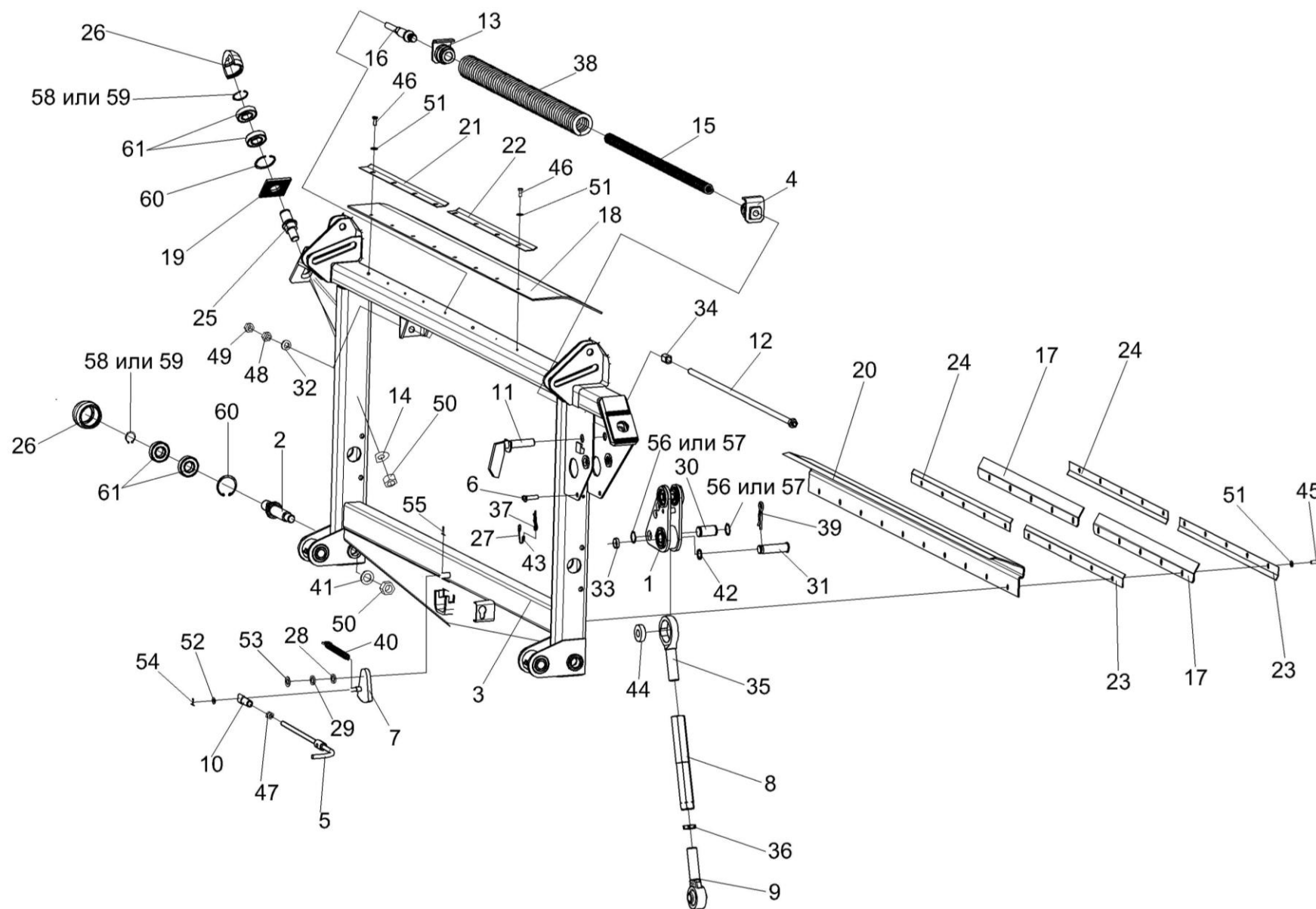
Рисунок 26а – Рамка переходная КЗК-9-1808000
