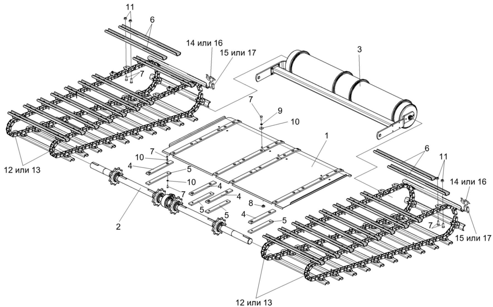
Рисунок 12а – Установка транспортеров КЗК-12-1817000Б
