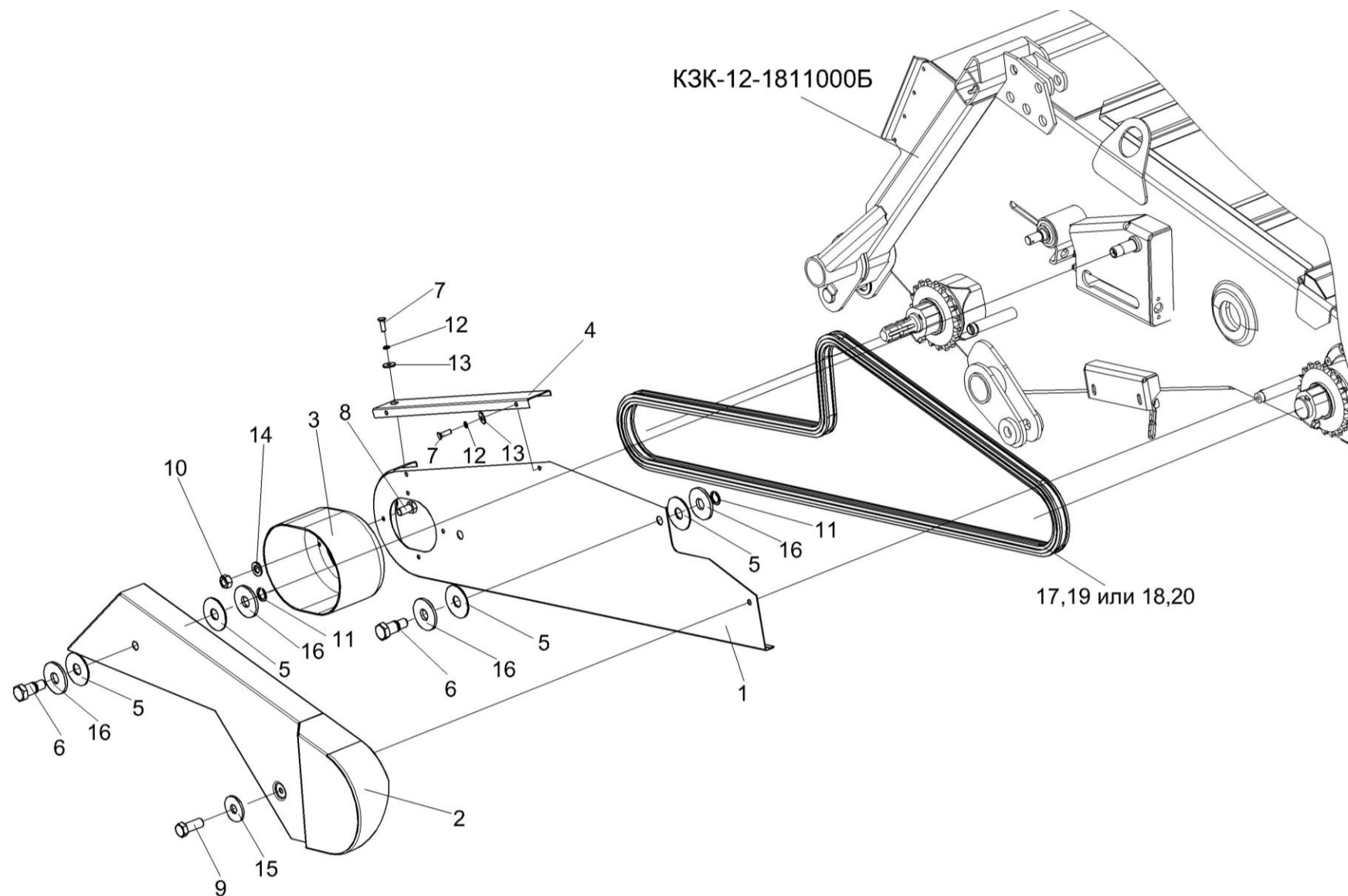
Рисунок 17а – Установка ограждений КЗК-12-1800140 и КЗК-12-1800160
