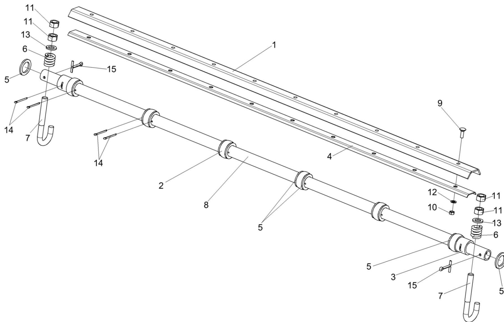
Рисунок 16а – Установка трубы КЗК 1770010-01
