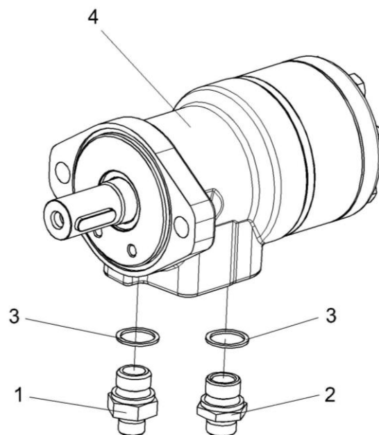
Рисунок 21а – Гидромотор КЗК-12-1790990А
