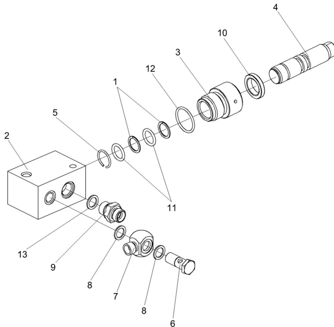
Рисунок 20а – Гидроцилиндр КЗК-12-1790200А
