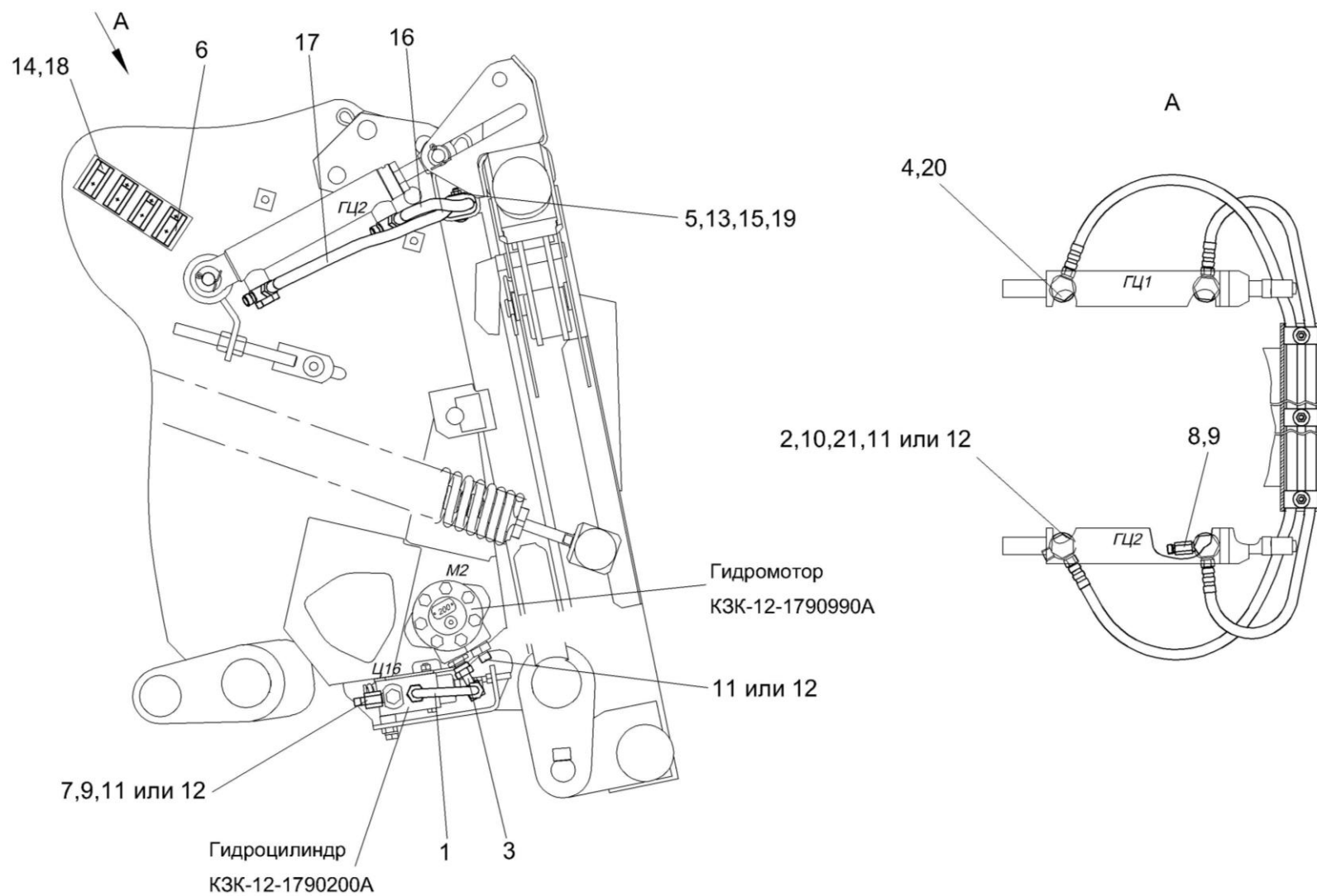
Рисунок 28а – Система гидравлическая камеры наклонной КЗК-12-1790000А
