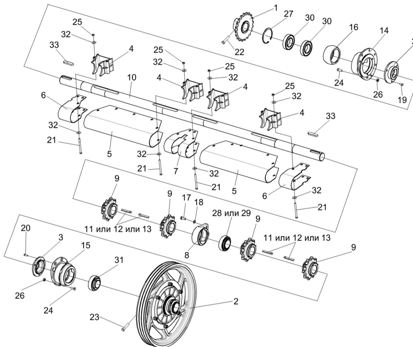
Рисунок 14а – Установка вала верхнего КЗК-12-1813000А
