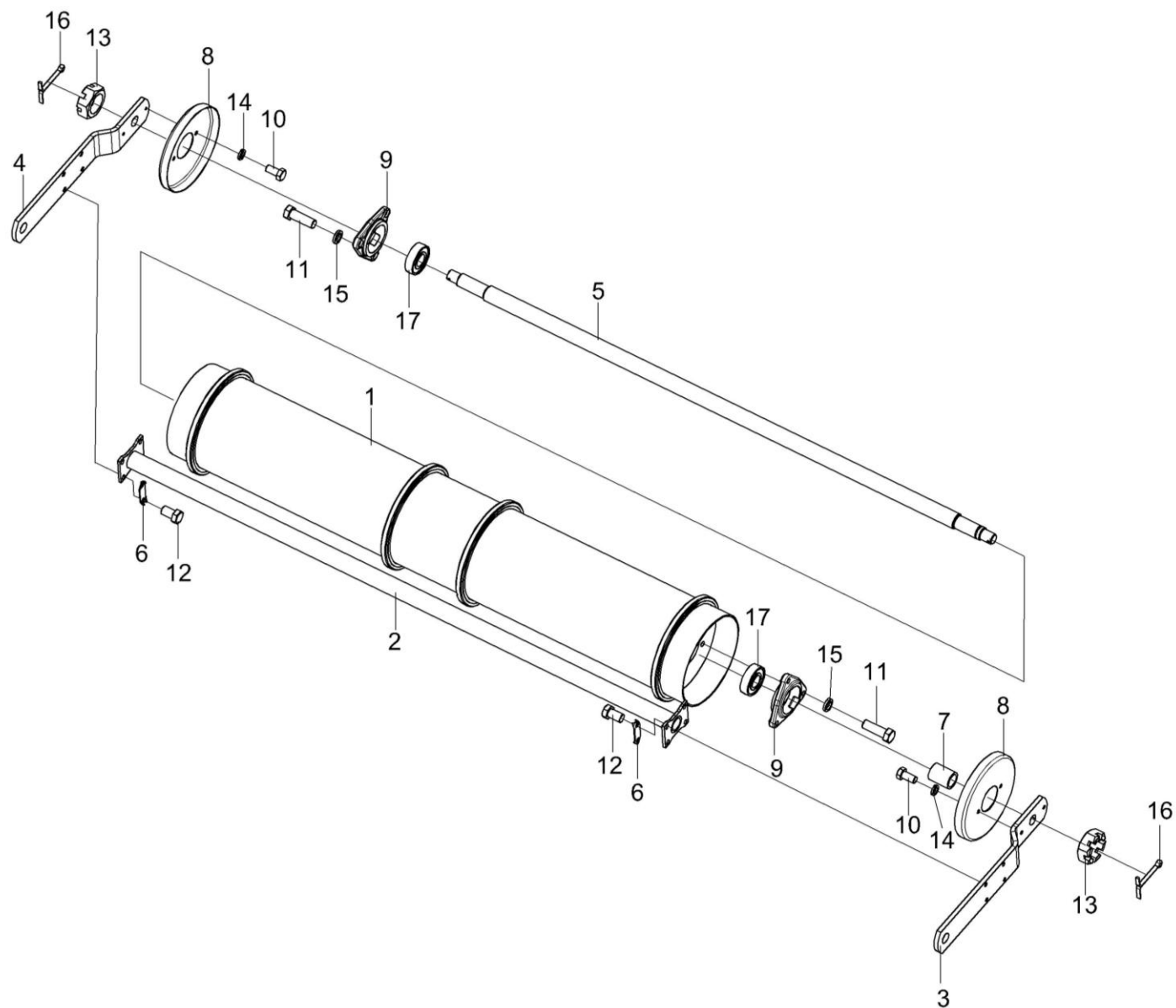
Рисунок 23а – Установка вала нижнего КЗК-12-1816000Б
