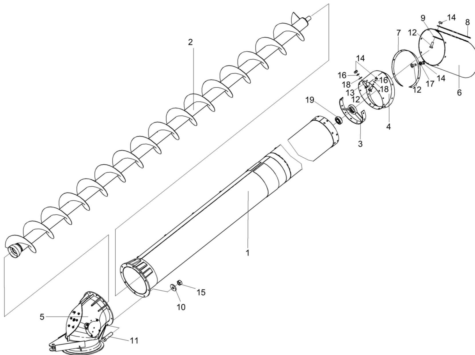
Рисунок 109а – Шнек с отводом КЗК-12-0206000А-01
