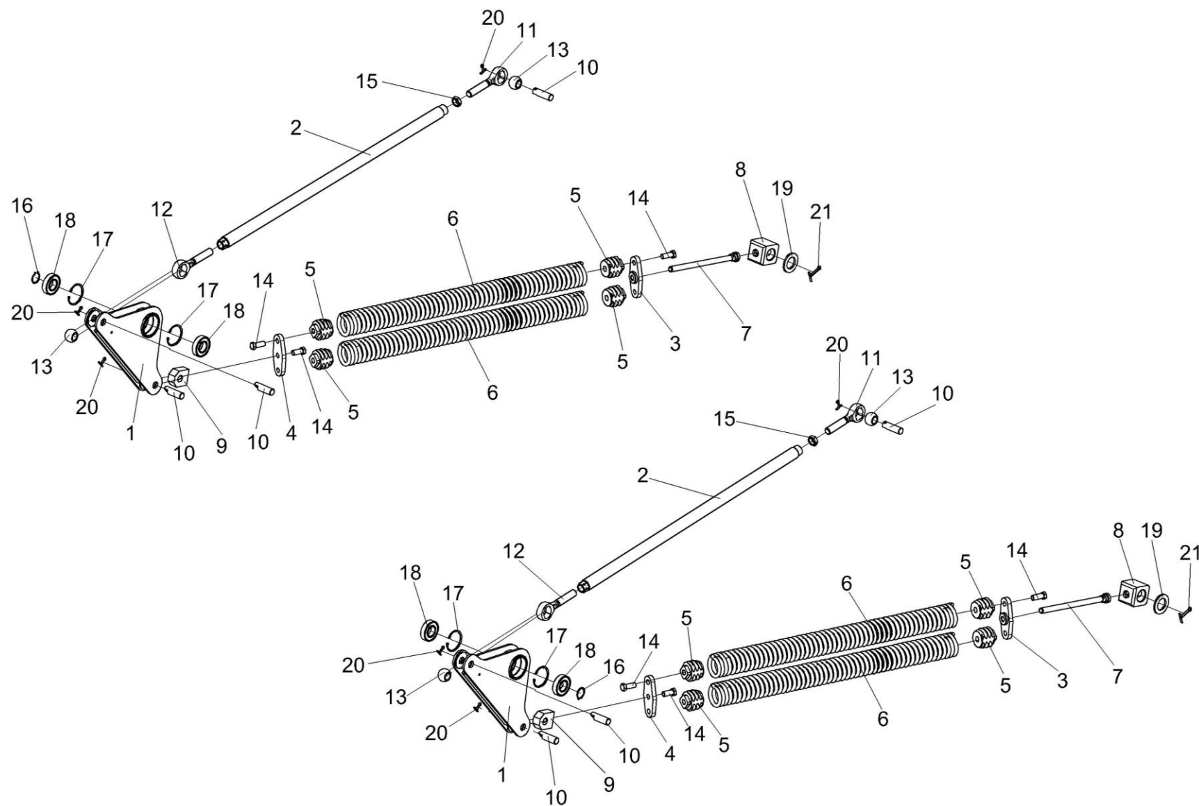
Рисунок 22а – Механизм продольного копирования КЗК-9-1805000
