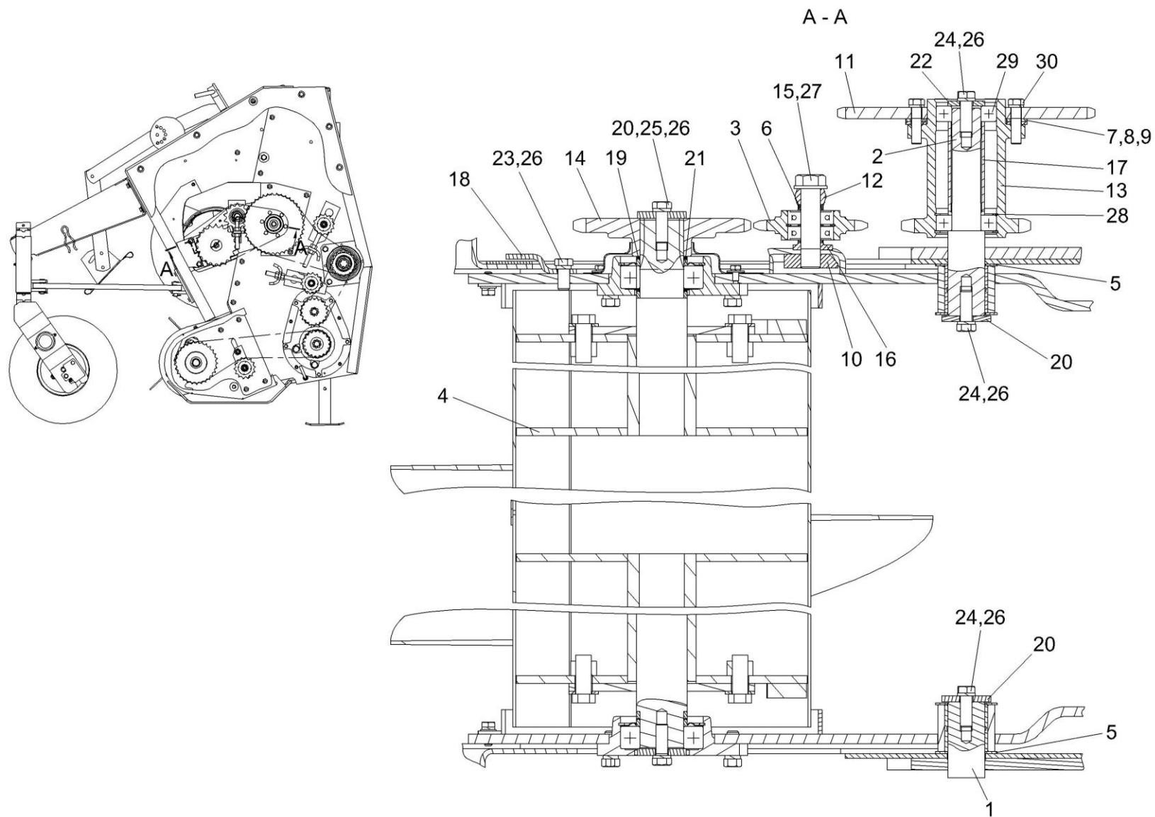
Рисунок 3 – Подборщик КВС-4-3900000 (вид сбоку) (лист 3)
