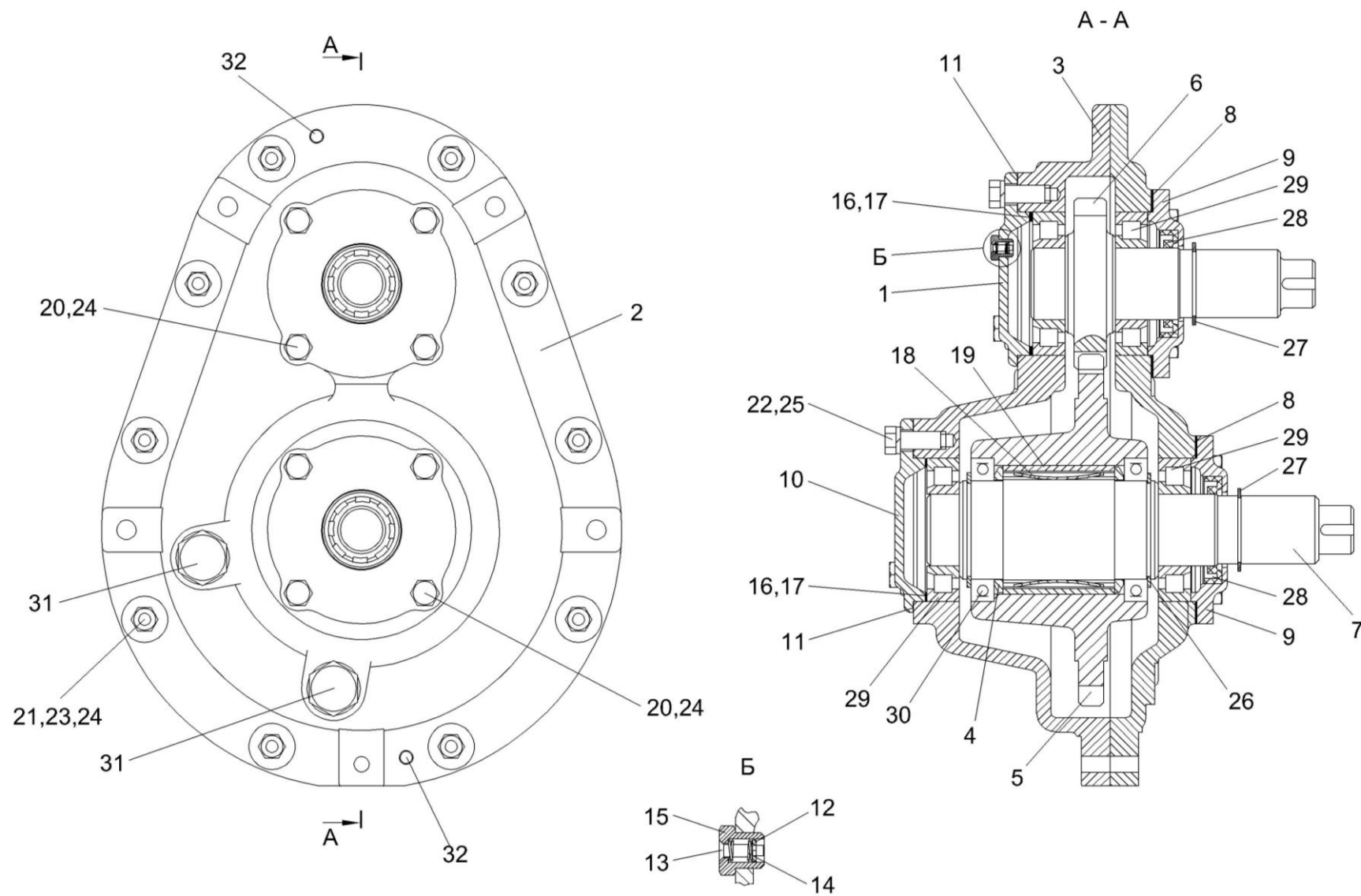
Рисунок 20 – Редуктор КВС-4-3904000
