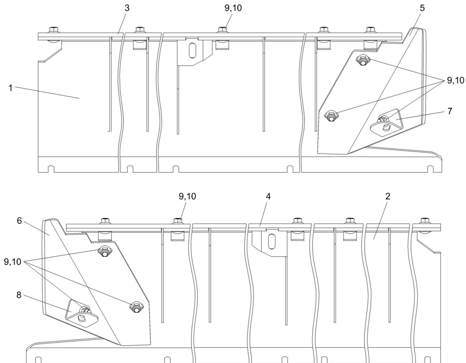
Рисунок 15 – Поддоны КВС-4-3901070 и КВС-4-3901080
