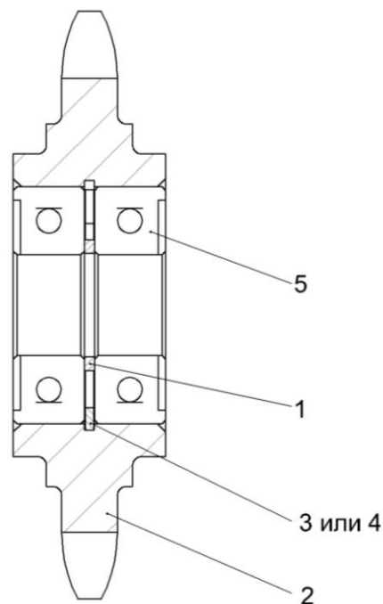
Рисунок 13 – Звездочка КВС-4-3900410
