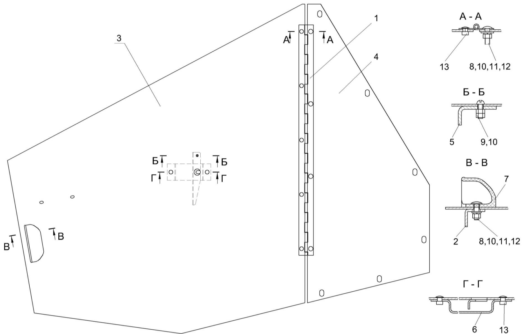
Рисунок 10 – Ограждение КВС-4-3900070
