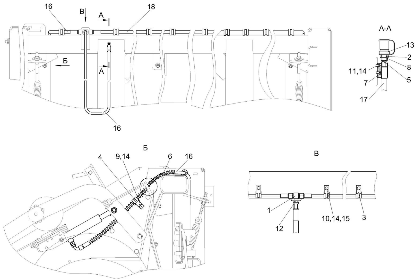
Рисунок 25 – Гидросистема подборщика КВС-4-3912000-01
