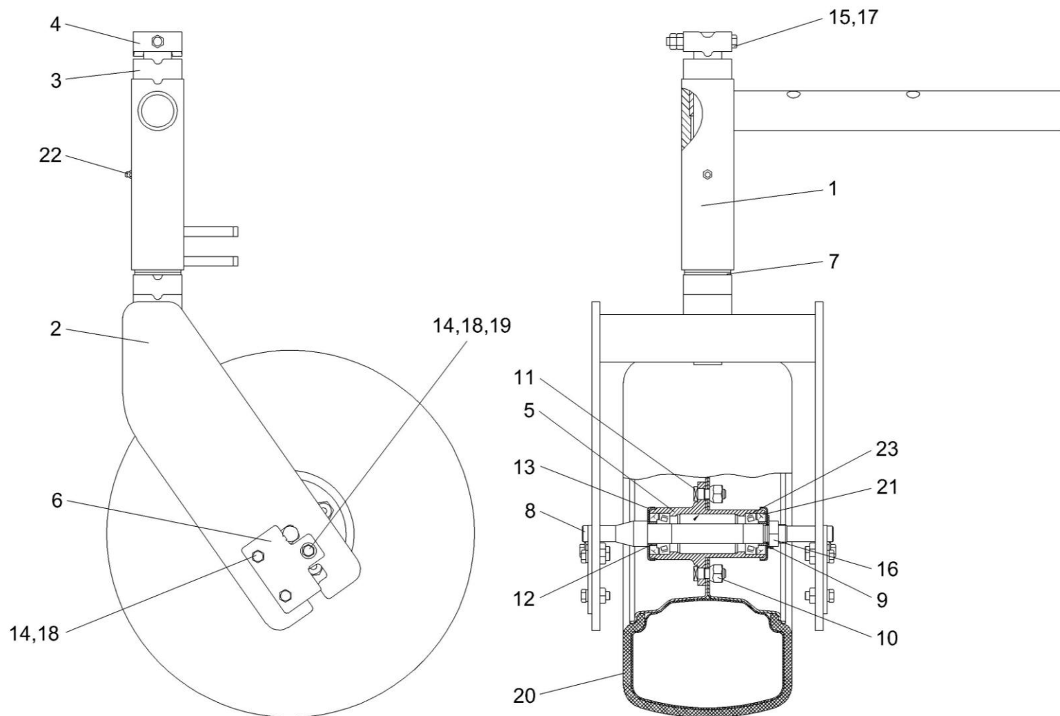
Рисунок 22 – Колесо флюгерное КВС-4-3920100 (изображено) Рисунок 23 – Колесо флюгерное КВС-4-3920100-01 (зеркальное отражение)
