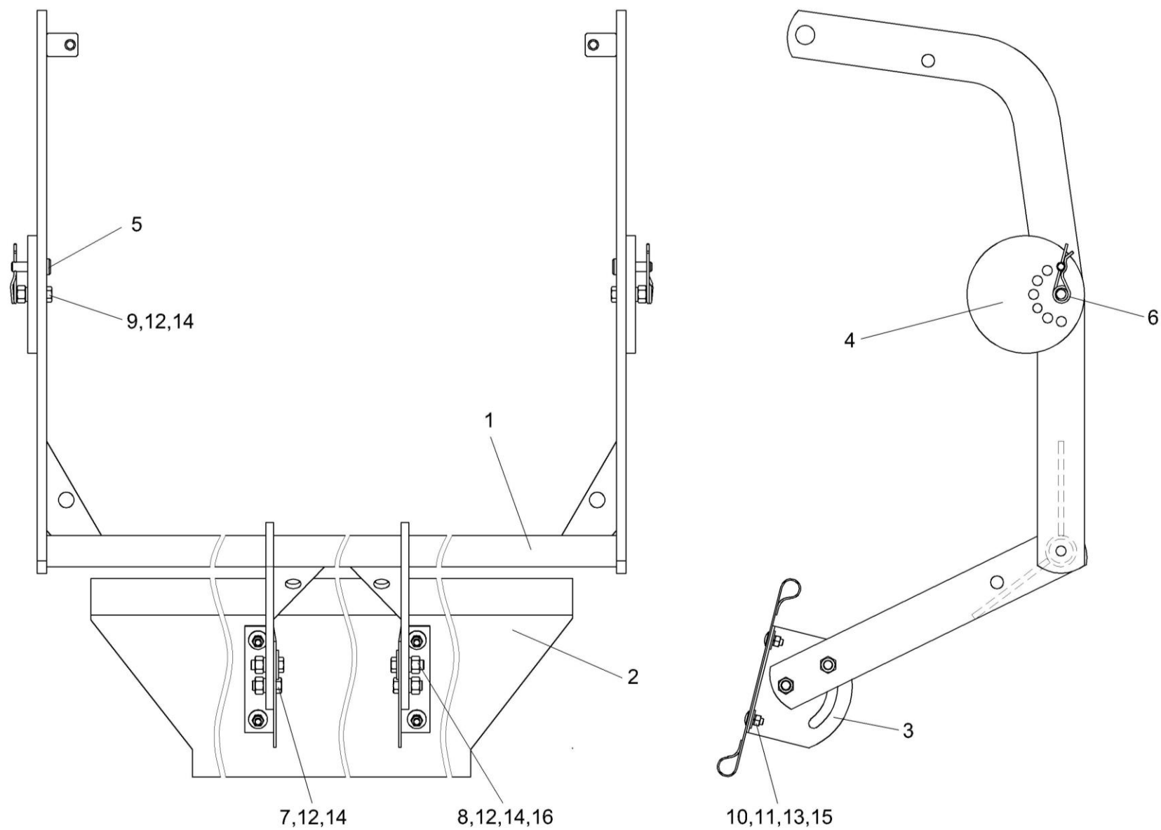
Рисунок 21 – Рамка прижимная КВС-4-3909000
