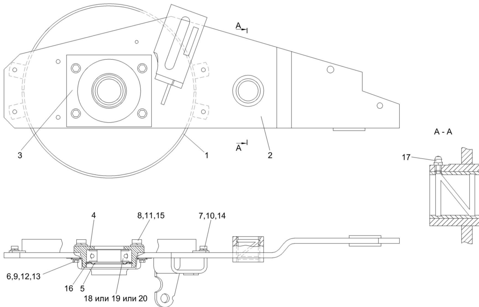
Рисунок 18 – Рычаг КВС-4-3902070А
