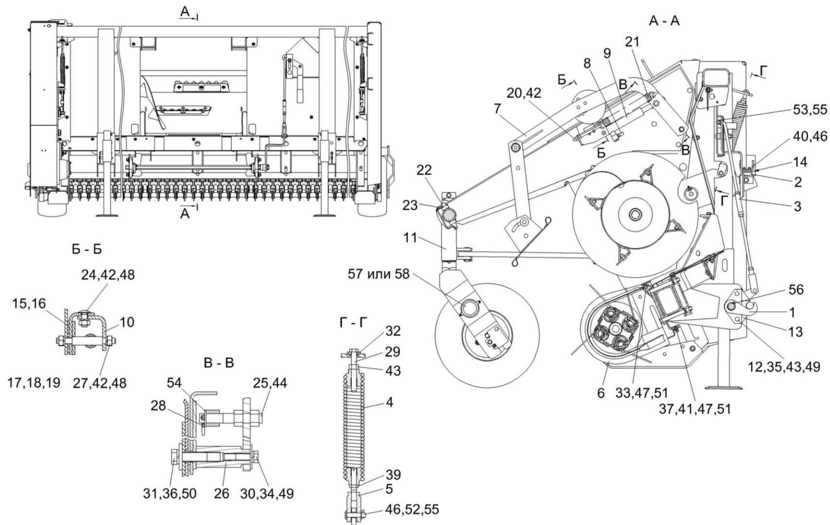
Рисунок 7 – Подборщик КВС-4-3900000 (вид спереди) (лист 2)
