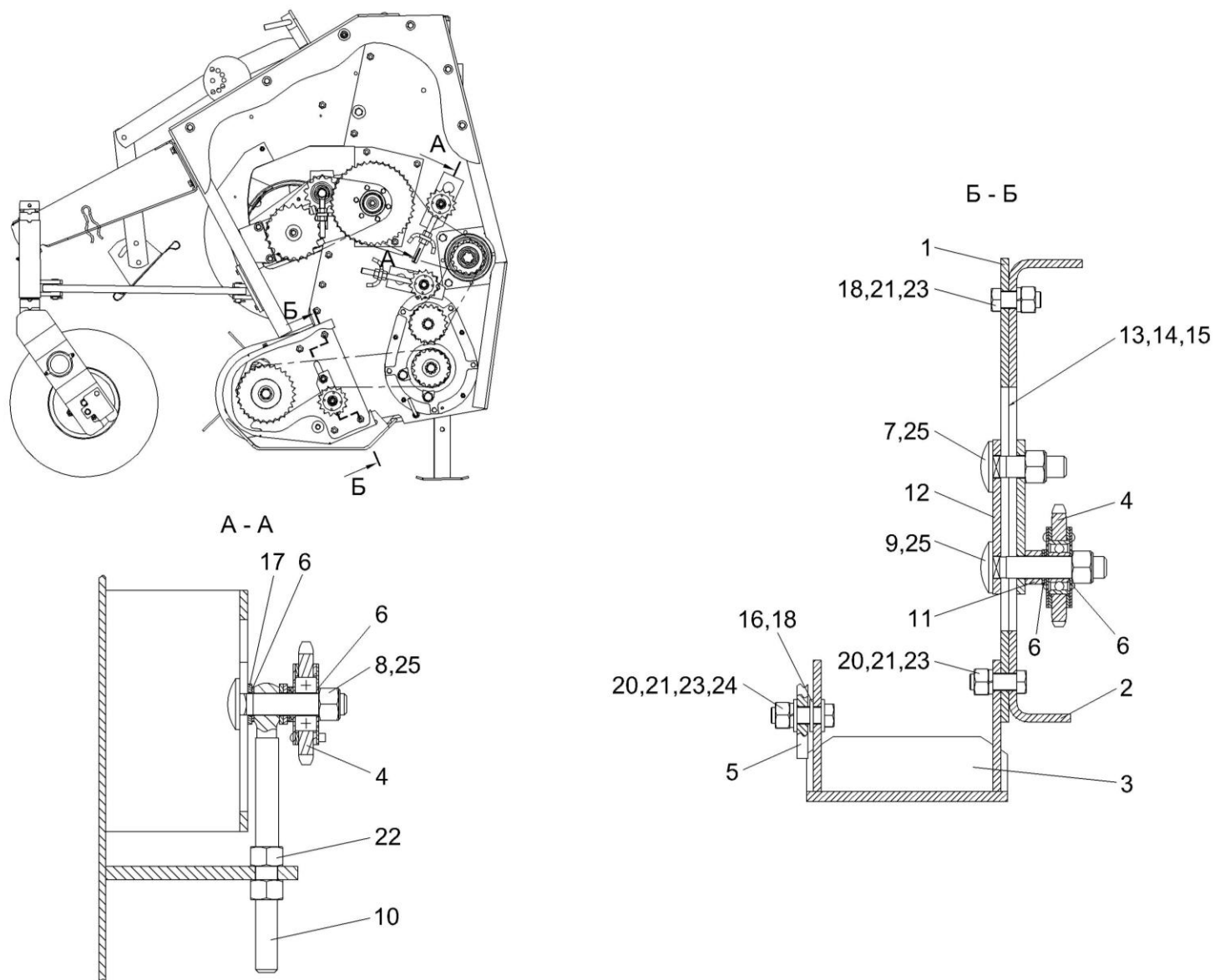
Рисунок 4 – Подборщик КВС-4-3900000 (вид сбоку) (лист 4)
